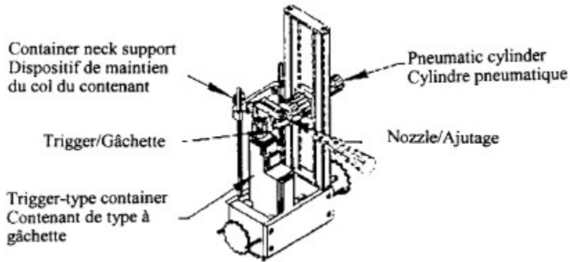
FIGURE 3 Appareil de maintien pour contenant de type à gâchette Vue isométrique
